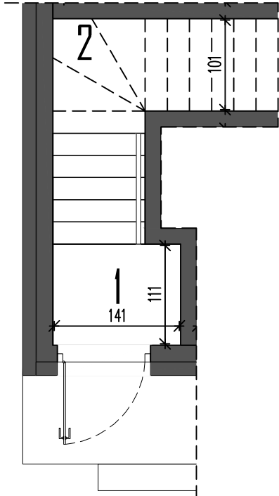
RZUT PARTERU
