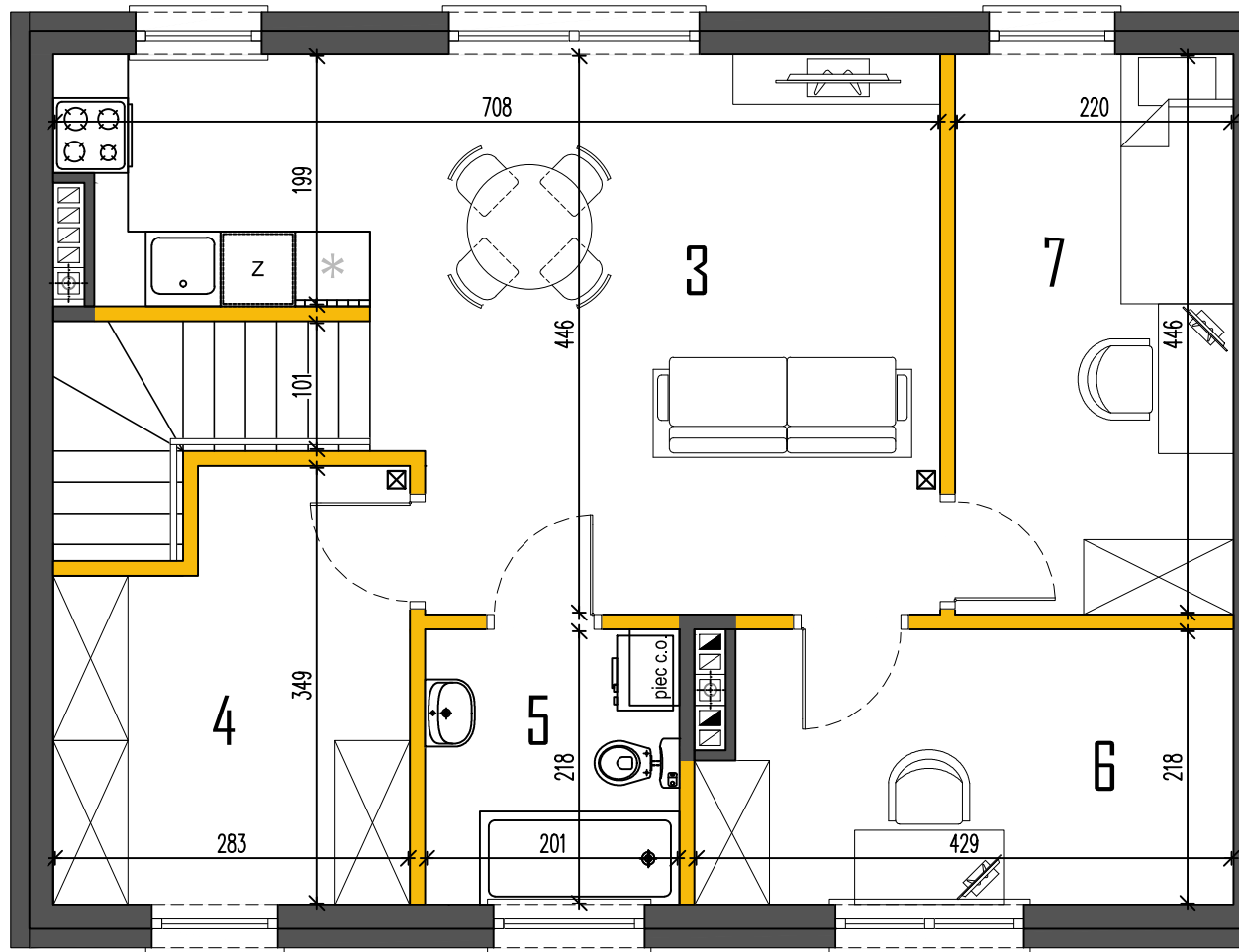
RZUT PIĘTRA
