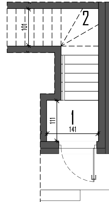
RZUT PARTERU
