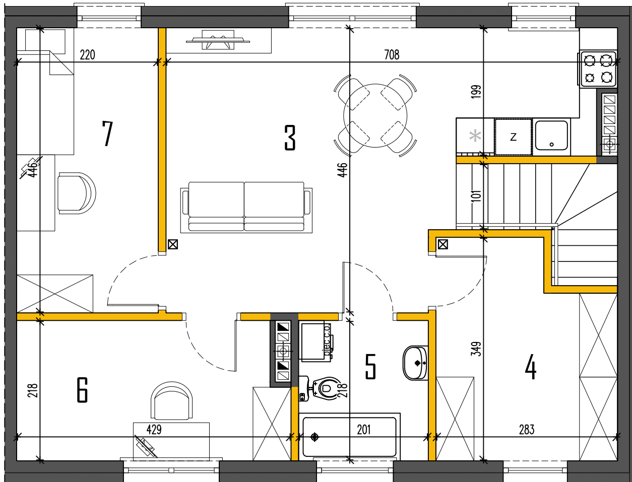
RZUT PIĘTRA
