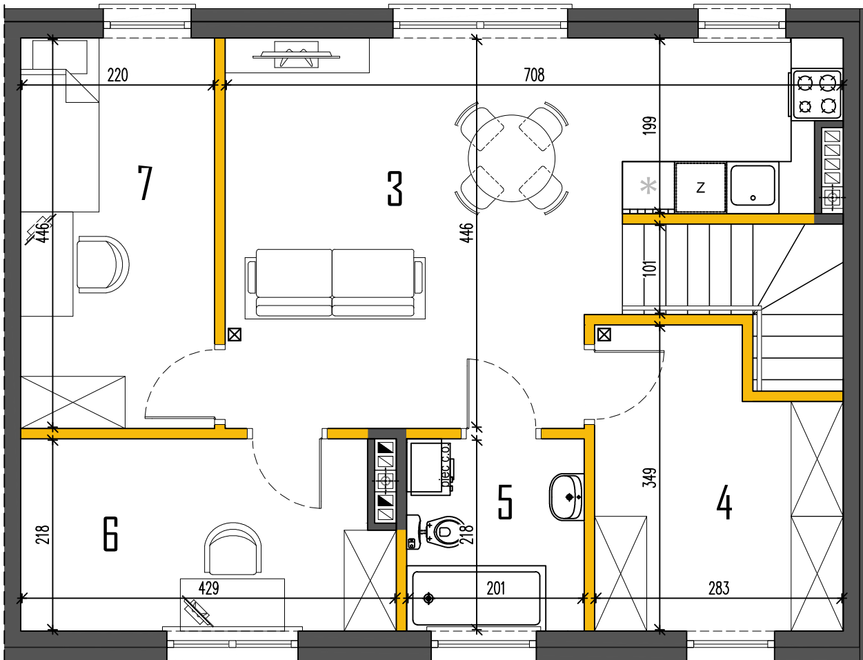
RZUT PIĘTRA
