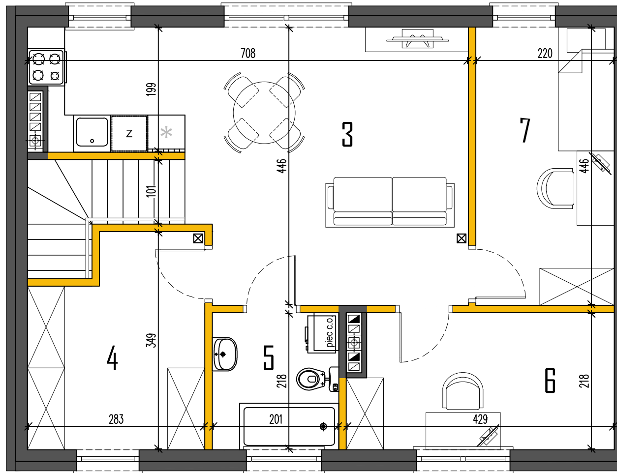
RZUT PIĘTRA
