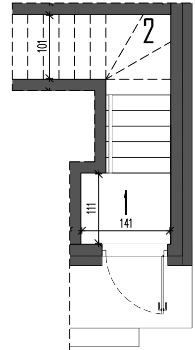
RZUT PARTERU
