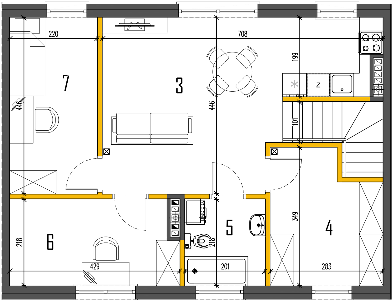
RZUT PIĘTRA
