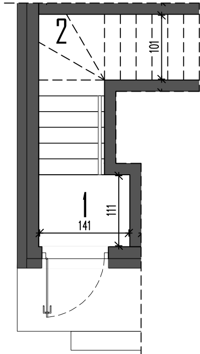
RZUT PARTERU
