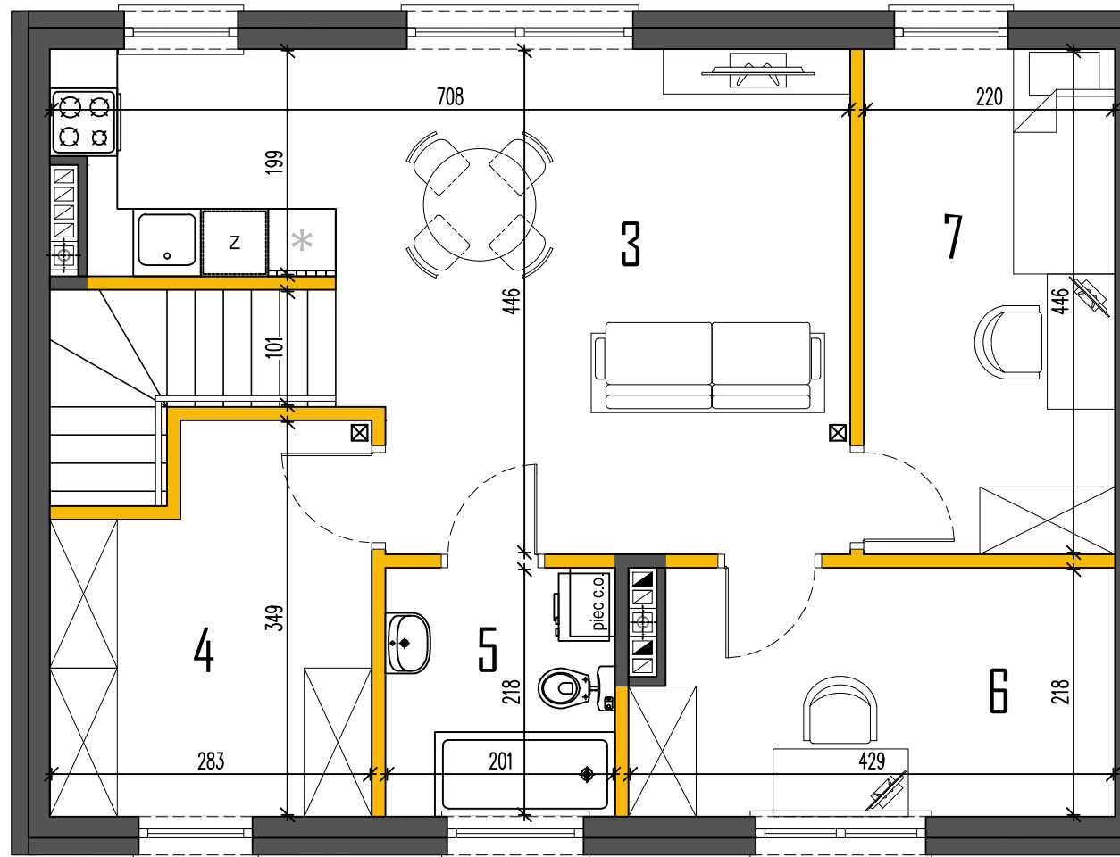
RZUT PIĘTRA
